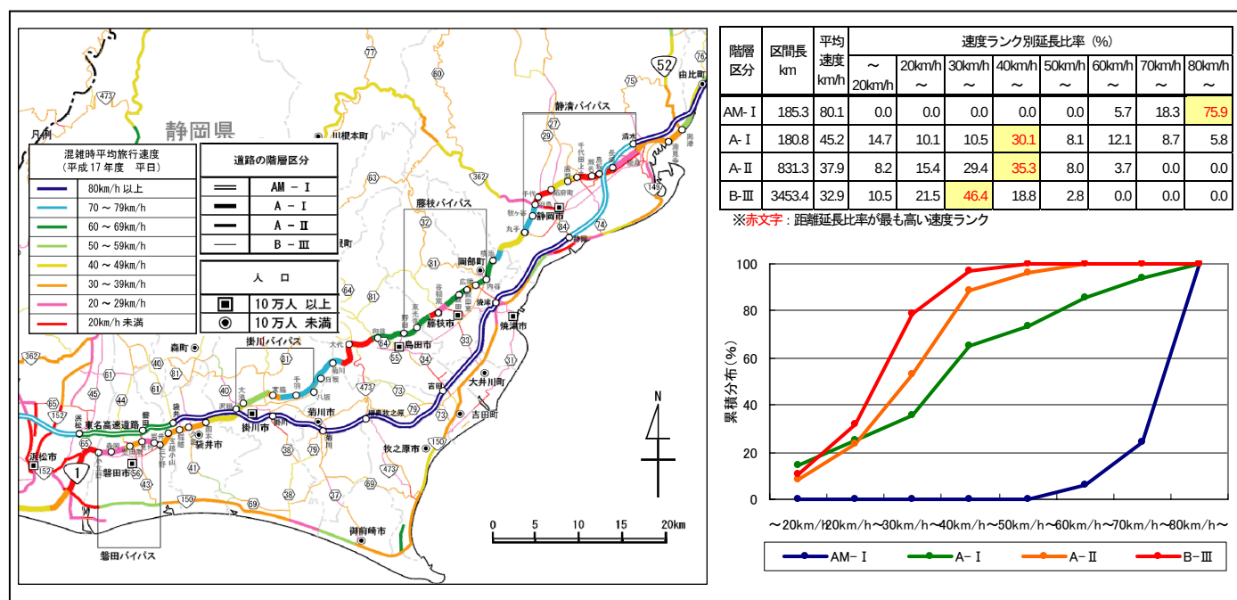
図-3 対象フィールドにおける道路の階層区分と速度水準(静岡県静岡市～浜松市の例)
