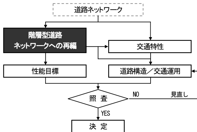
図－2 性能照査型道路計画設計の流れ
