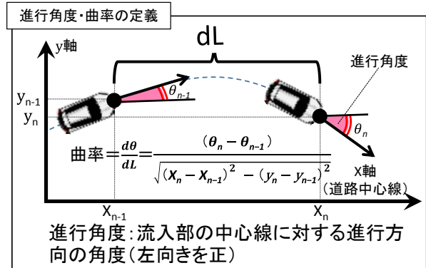
図-2 曲率と進行方向角の定義
