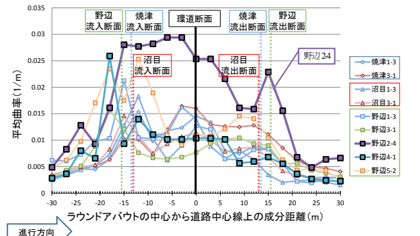
図-9 曲率の標準偏差のプロファイル
